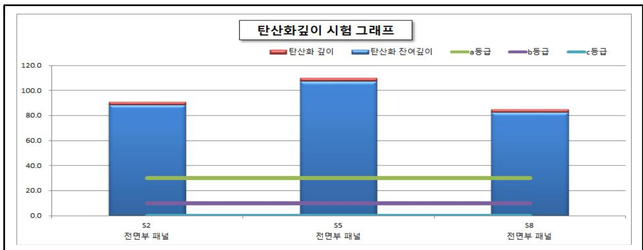
【그림 5.4.3】 탄산화 깊이 측정결과
